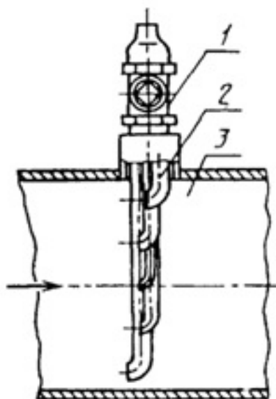
Рис. 1.1. Схема отбора проб из скважины с помощью зонда
