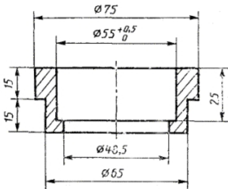
Пробка
