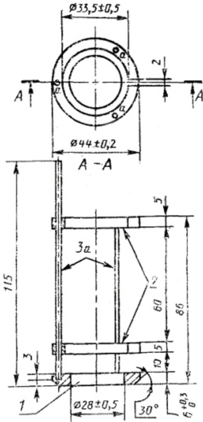
Поддержка кольца; 2 - прокладки; 3a - проволоки из нержавеющей стали
